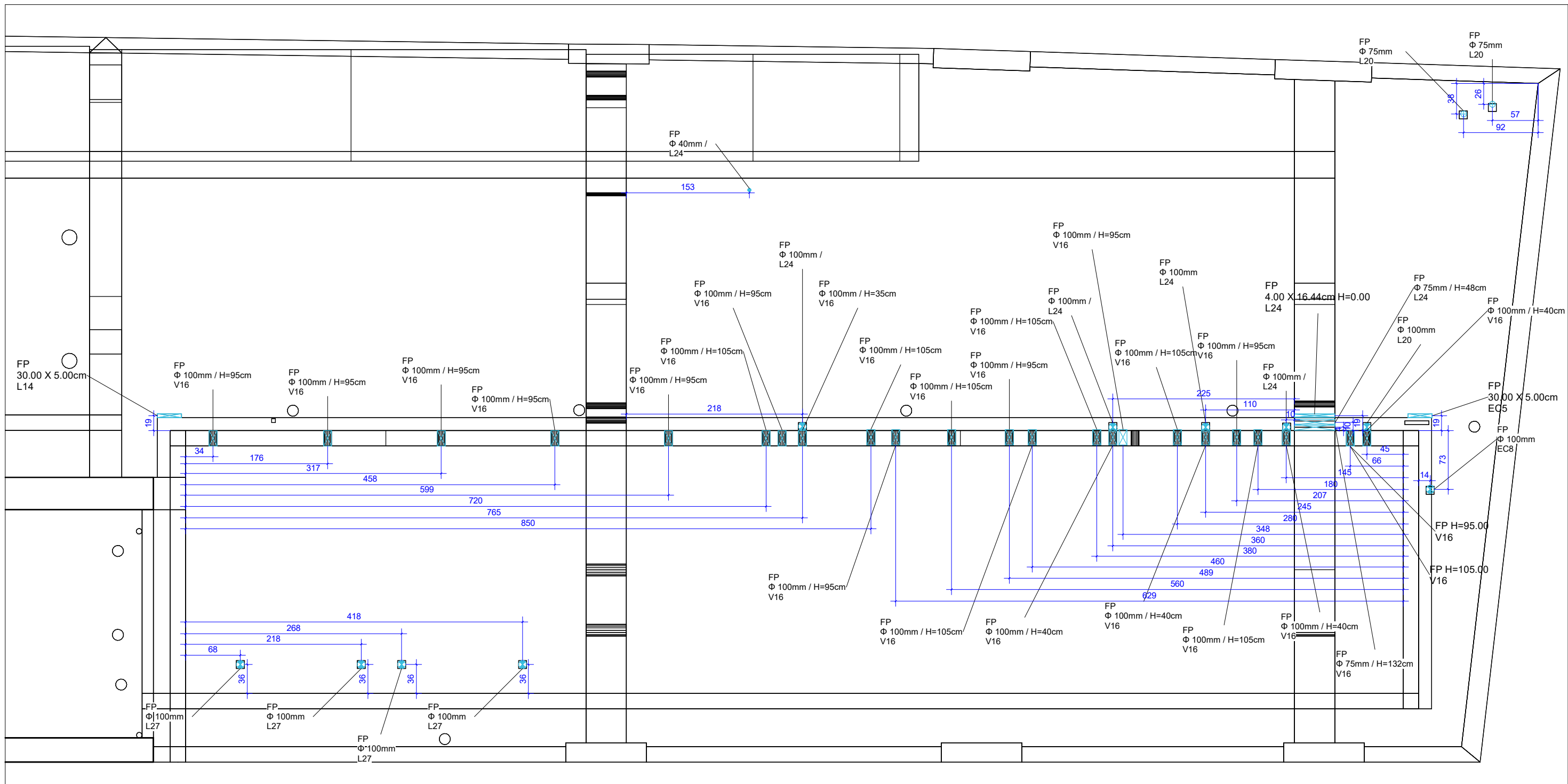
PAVTO. LAZER - MARCAÇÃO FUROS ESCALA 1:50
