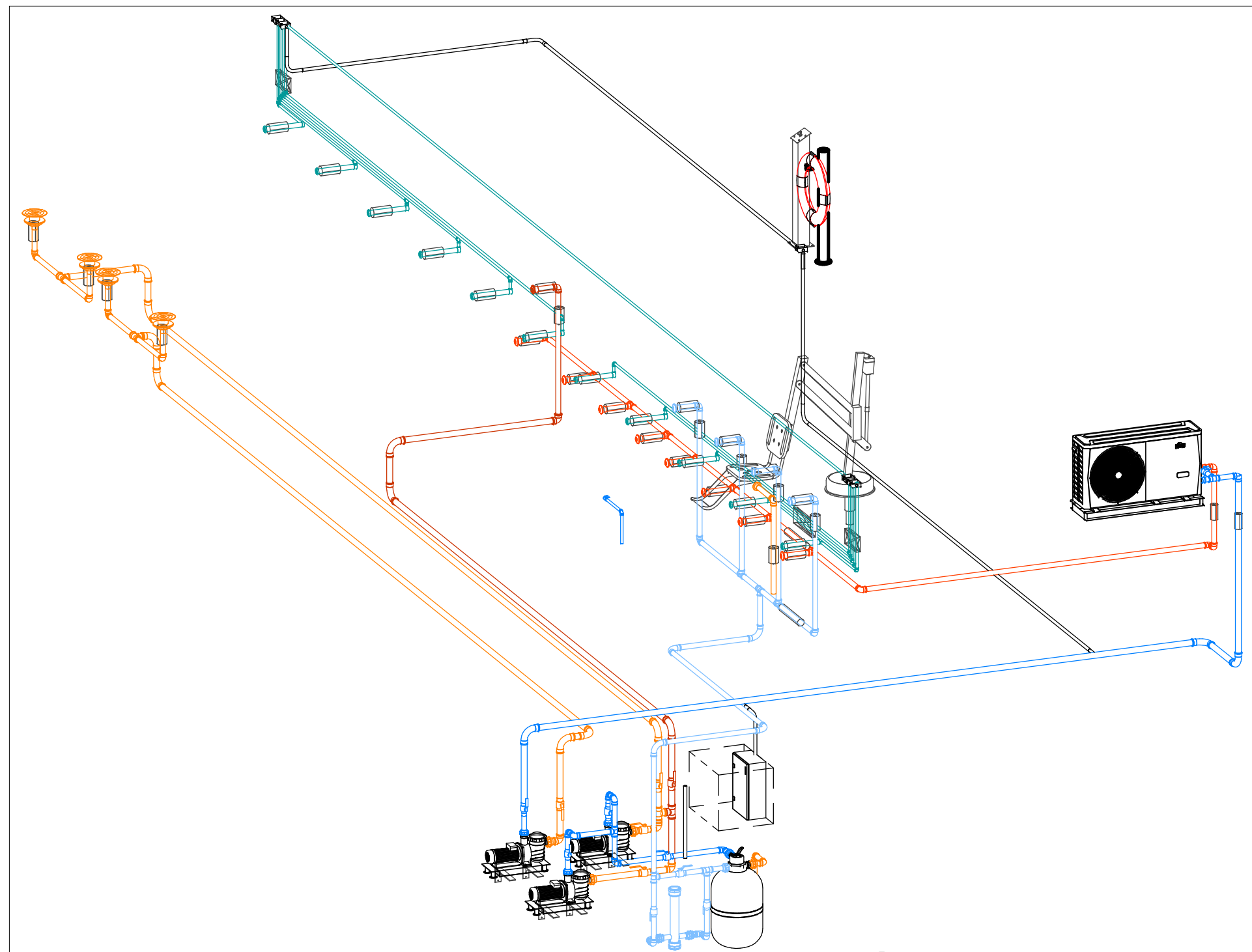
ISOMÉTRICO REDE PISCINA ESCALA 1:50
